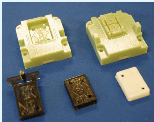
3Dプリンターで作った樹脂製の「金型」
